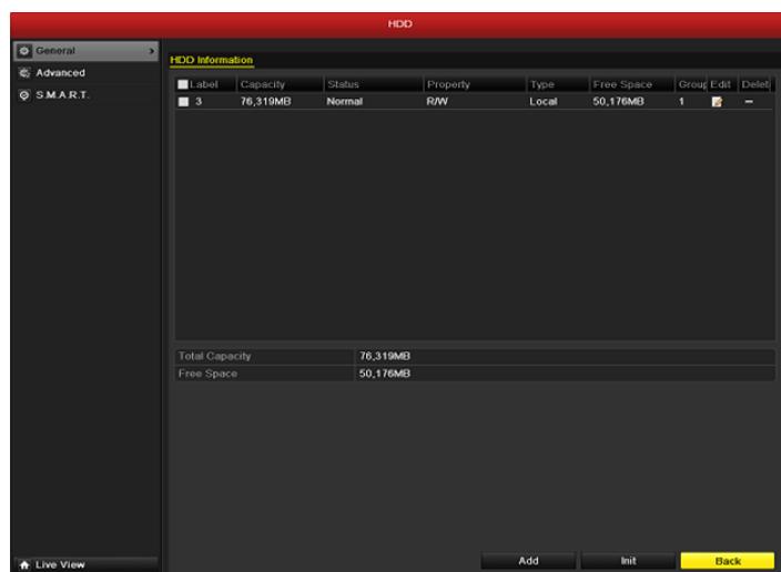
Obr. 5.1 HDD - Všeobecně
