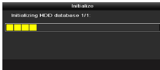
Obr. 10.3 Spuštění inicializace
