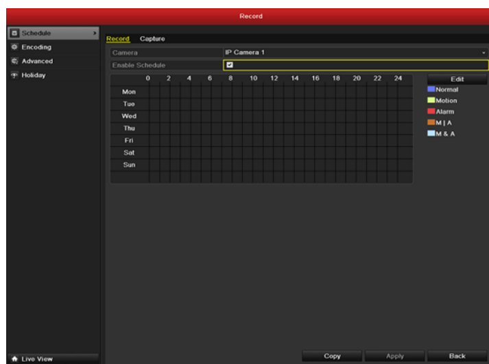
Obr. 5.29 Rozvrh záznamu
