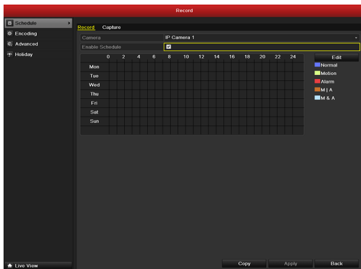
Obr. 5.14 Rozvrh záznamu
