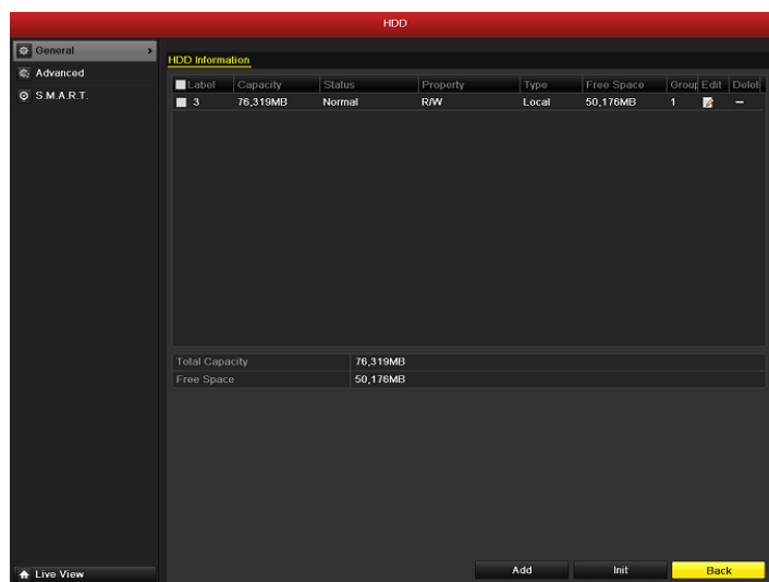
Obr. 5.40 HDD všeobecně
