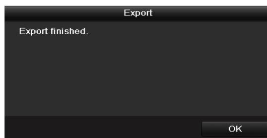
Obr. 7.34 Ukončení exportu
