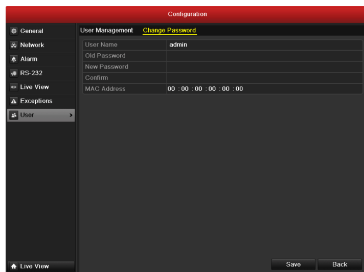
Obr. 13.12 Změna hesla
