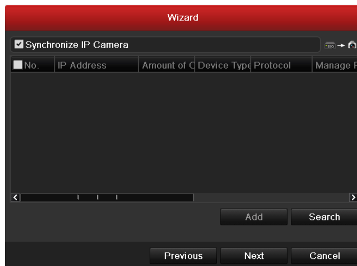
Obr. 2.6 Nastavení záznamu
