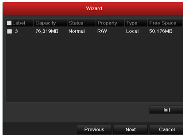
Obr. 2.5 Správa HDD
