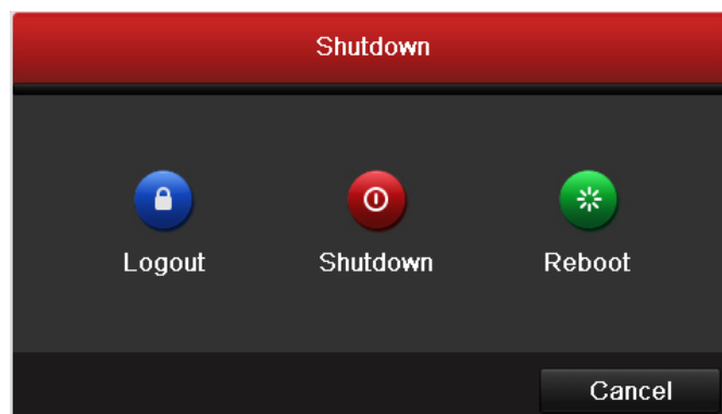
Obr. 3.9 Menu vypínání
