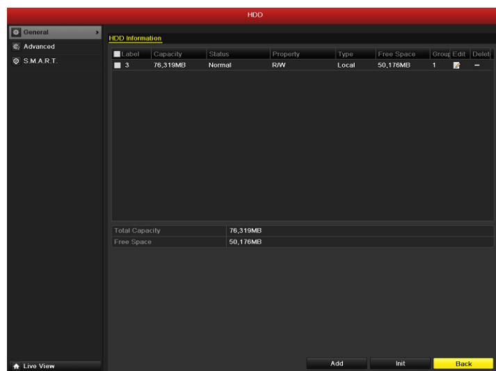
Obr. 5.31 HDD všeobecně
