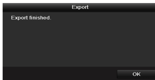
Obr. 7.29 Ukončení exportu
