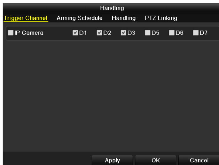
Obr. 5.21 Zpracování poplachu
